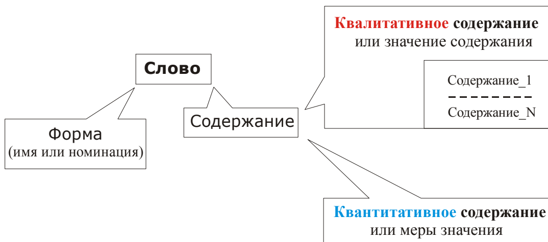
Рис.2. Граф слова.
